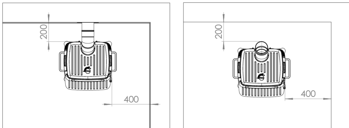
Figure 3 (distances face aux parois en matériau ininflammable)
