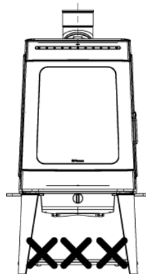
Figure 2 (distances face aux parois en matériau combustible)
