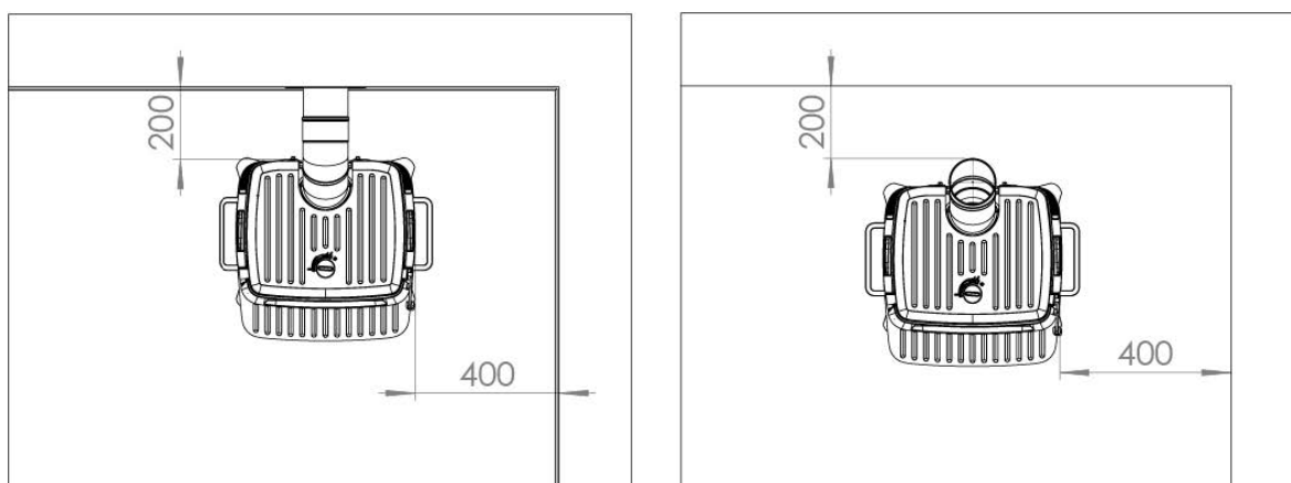
Slika 3 (Razmak od nezapaljivog materijala)
