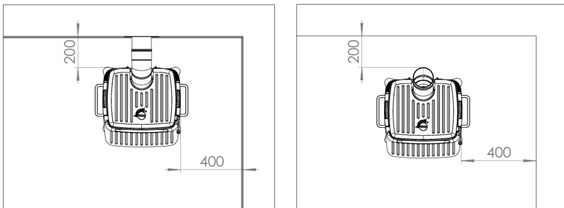
Abbildung 3 (Abstände zu Wänden aus nicht brennbarem Material)
