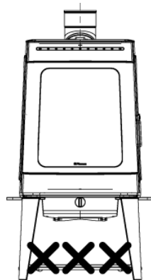
Abbildung 2 (Abstände zu Wänden aus brennbarem Material)
