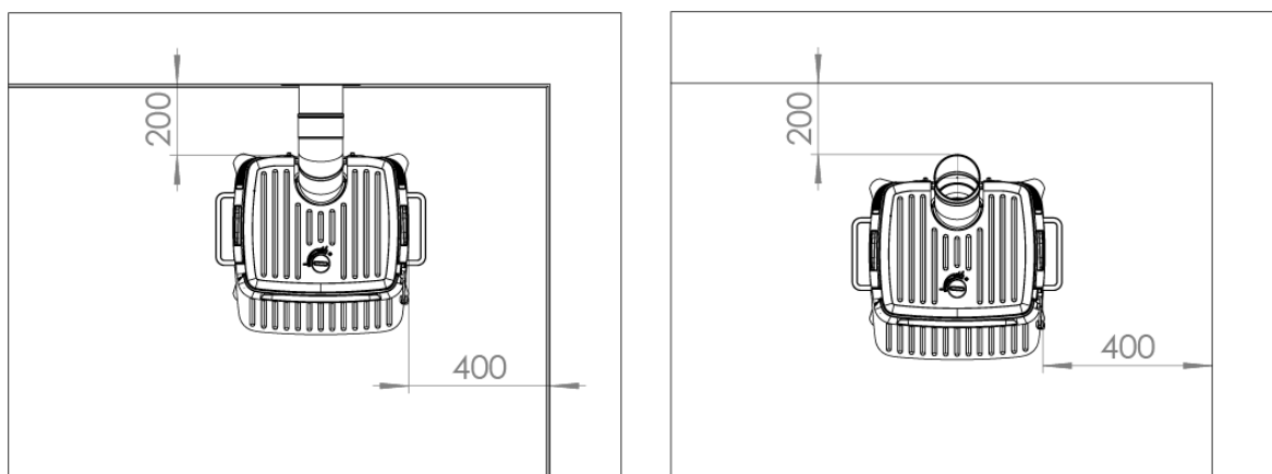
Figura 3 (distanza da materiale non infiammabile)
