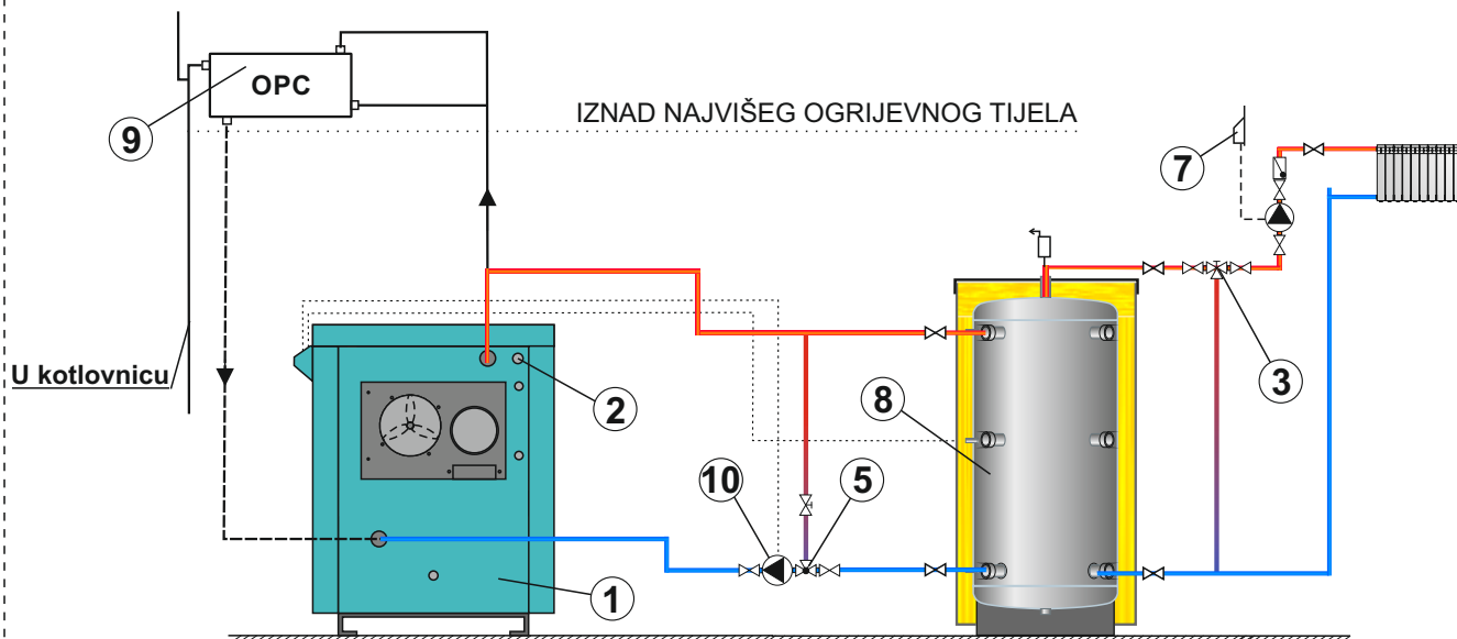
Shema 3a. Primjer kada je prema EN 303-5 potrebna ugradnja akumulacijskog spremnika u sustav centralnog grijanja
