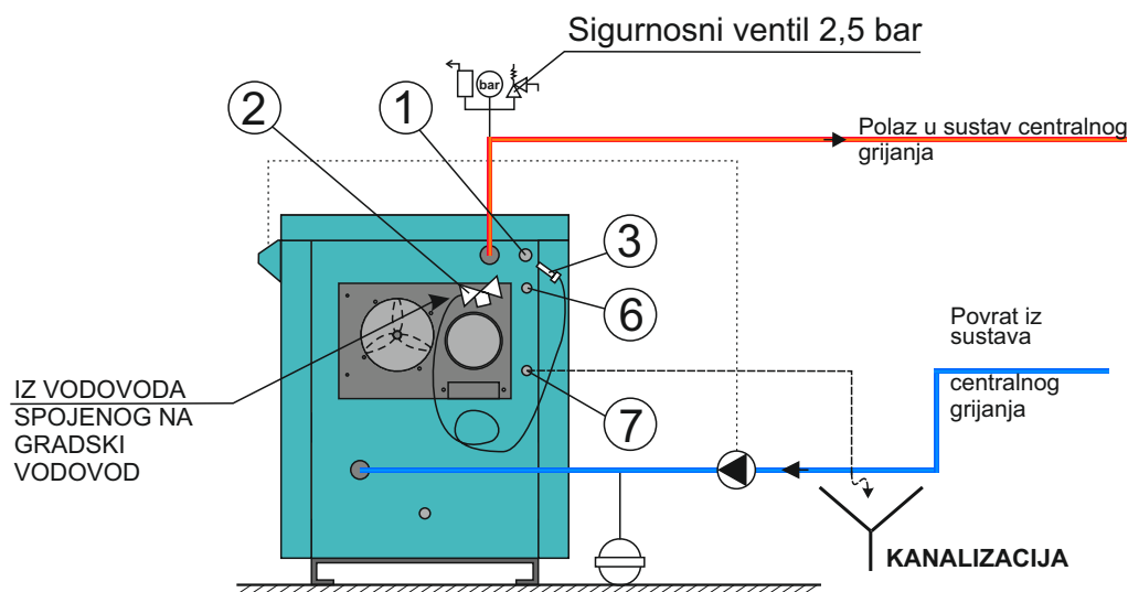
Shema 2. Prikaz ugradnje termičke zaštite kotla BioSolid ugrađenog na zatvoreni sustav grijanja
