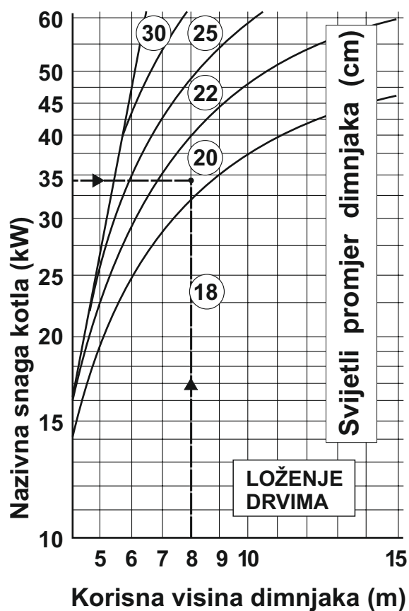
Slika 3. Dimenzioniranje dimnjaka za kotlove BioSolid
